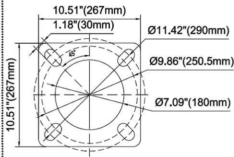
7" Flange
