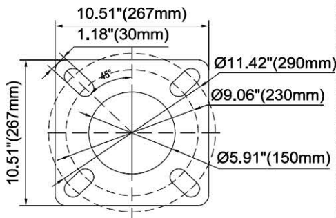
6" Flange
