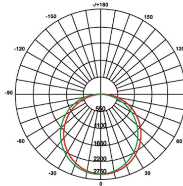
2PT-80/100/120/150W-3CCT-PC 150W @ 5000K
